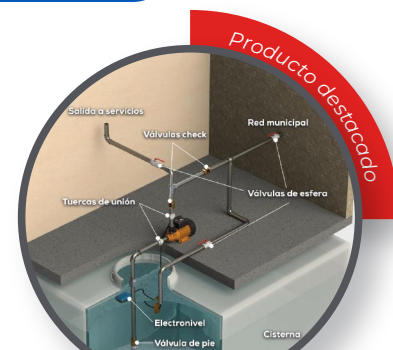
Bomba periférica 1/2" Hp BP1ME050 SKU: 0218030004
